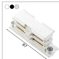
XTS21.(W, G, B) Jonction linéaire
